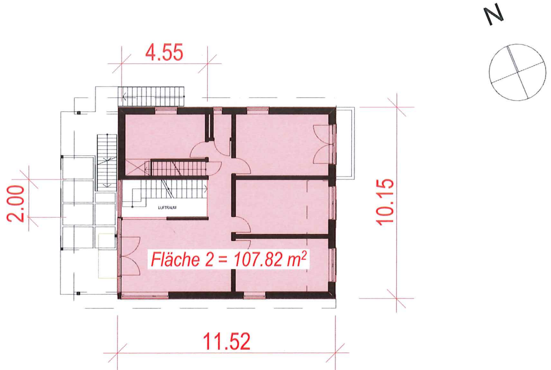
1.OBERGESCHOSS
