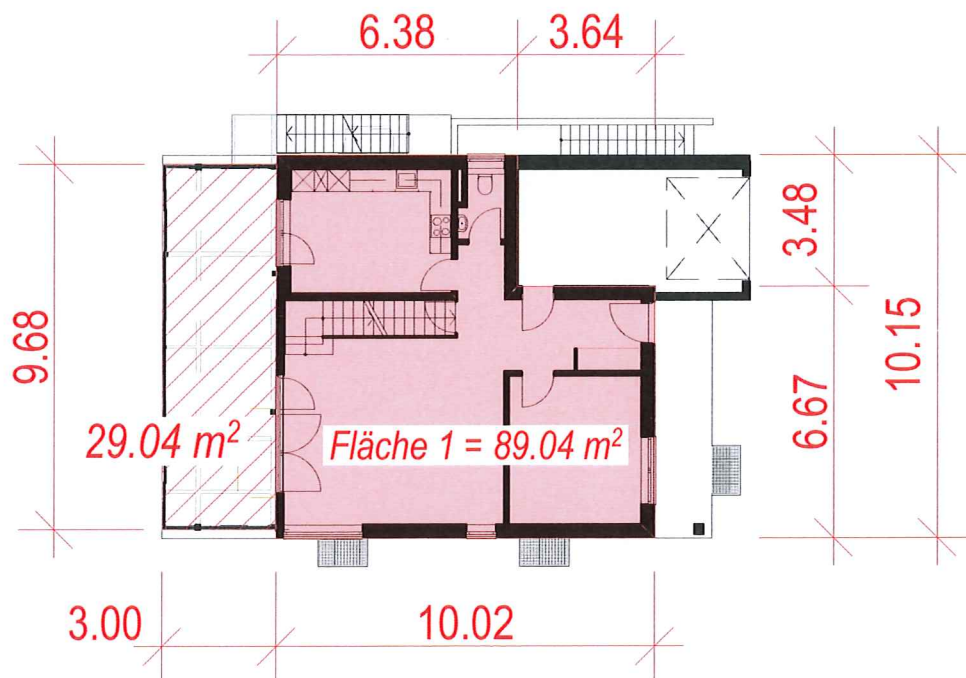
ERDGESCHOSS
